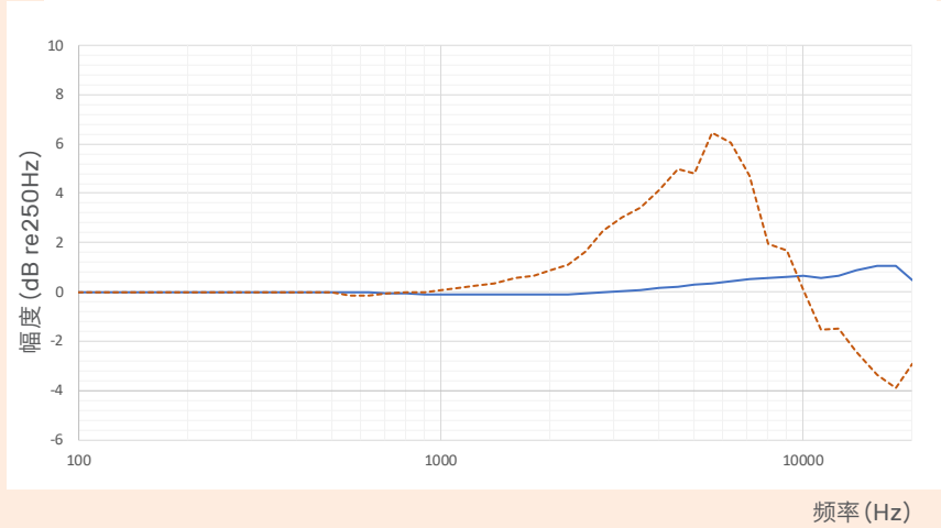
147EB 0度入射角典型的自由场频率响应
